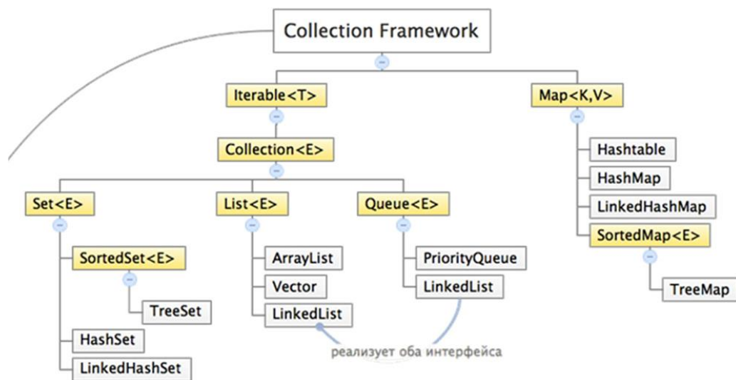
Рис. 3.1. Ієрархія інтерфейсів JCF і їх реалізацій
